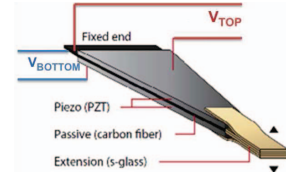
(b) Bimorph Actuator
